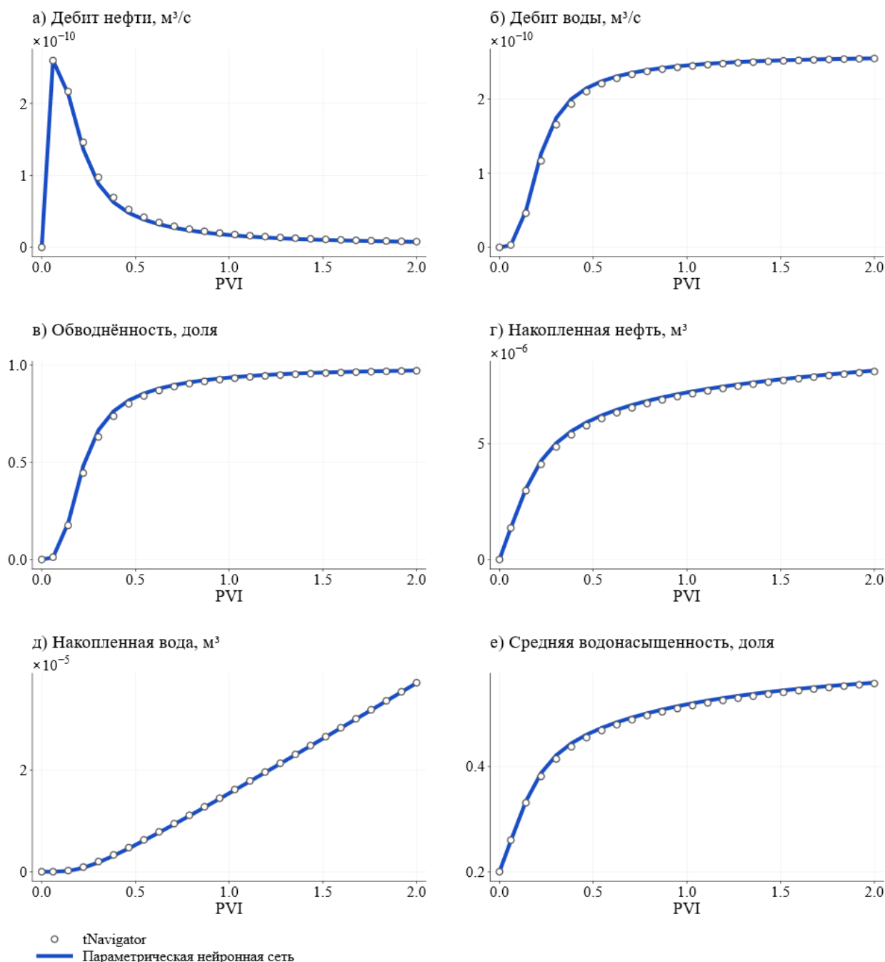
Рис. 2. Характеристики вытеснения в режиме q100. Незакрашенные кружки — tNavigator; синяя сплошная линия — параметрическая PINN
