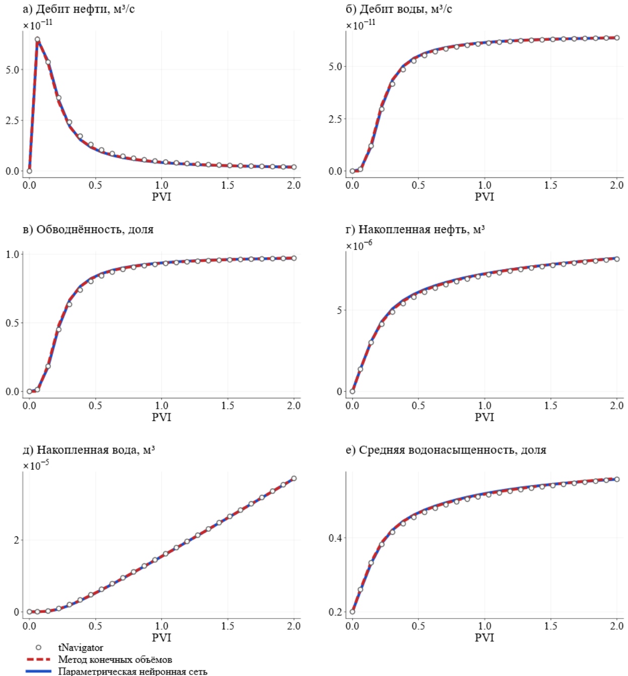
Рис. 1. Характеристики вытеснения в режиме q025. Незакрашенные кружки — tNavigator; красная пунктирная линия — метод конечных объемов; синяя сплошная линия — параметрическая PINN
