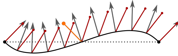
Рис. 2. Интерполяция нормали по методу Vlachos — красным, отражение средней нормали — оранжевым, истинная нормаль — серым
