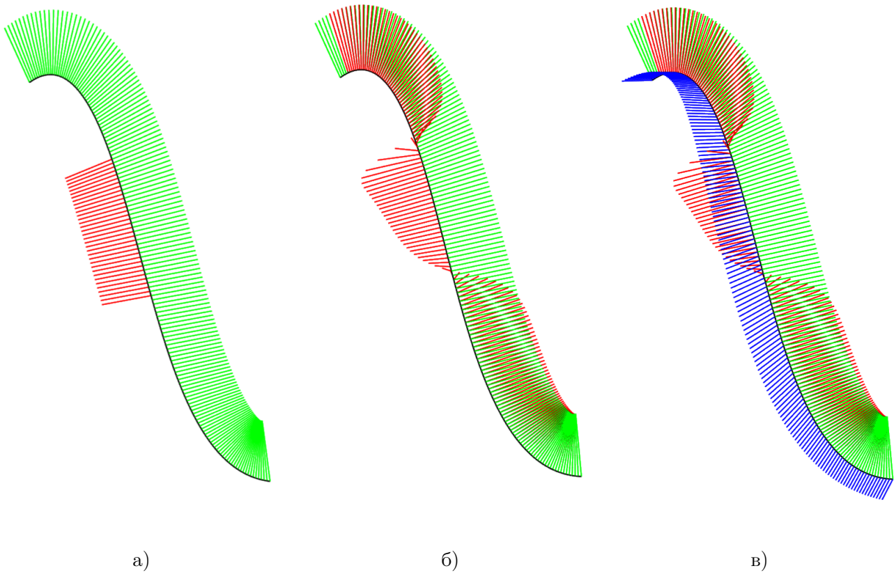
Рис. 13. Интерполяция нормали смешивающей функцией бинормалей (зеленым), смешивающей функцией нормалей вершин (красным), бинормаль (синим). а) случай плоской кривой; б–в) нормали в вершинах слегка смещены от общей плоскости; в) вид с бинормалью
