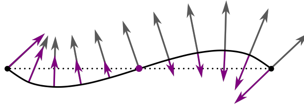
Рис. 9. Главная нормаль кривой, истинная нормаль — серым
