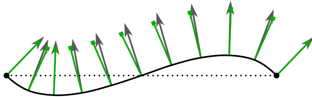
Рис. 4. Интерполяция нормали по методу Overveld–Wyvill — зеленым, истинная нормаль — серым
