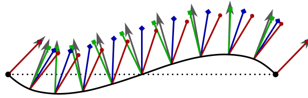
Рис. 5. Сравнение методов интерполяции нормали. Vlachos — красным, полином Бернштейна второй степени — синим, Overveld-Wywill — зеленым, истинная нормаль — серым
