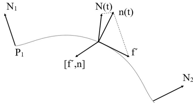
Рис. 10. Интерполяция нормали
