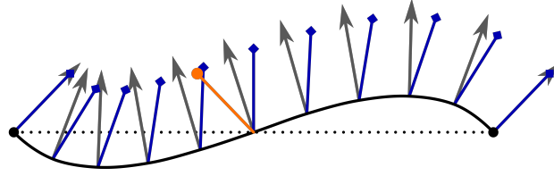
Рис. 3. Интерполяция нормали полиномом Бернштейна второй степени — синим, отражение средней нормали — оранжевым, истинная нормаль — серым
