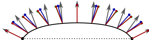
Рис. 7. Сравнение методов интерполяции нормали на выпуклой кривой. Vlachos — красным, полином Бернштейна второй степени — синим, Overveld-Wywill — зеленым, истинная нормаль — серым
