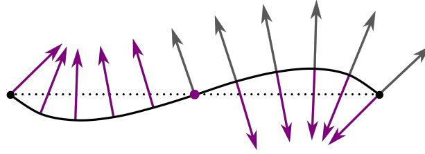
Рис. 8. Главная нормаль кривой (нормализованный вектор), истинная нормаль — серым
