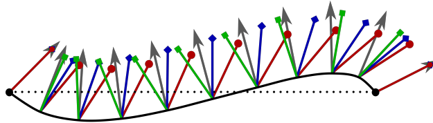
Рис. 6. Сравнение методов интерполяции нормали при другом направлении нормалей в вершинах. Vlachos — красным, полином Бернштейна второй степени — синим, Overveld-Wywill — зеленым, истинная нормаль — серым
