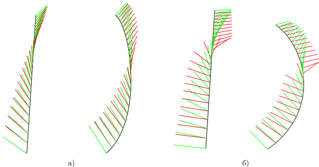
Рис. 14. Интерполяция нормали по кривой с экстремально развернутыми нормальными векторами вершин (формулой Родрига — зеленым, линейной функцией — красным)
