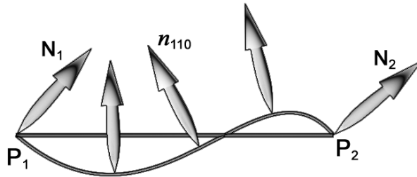
Рис. 1. Заявленная интерполяция нормали [1]
