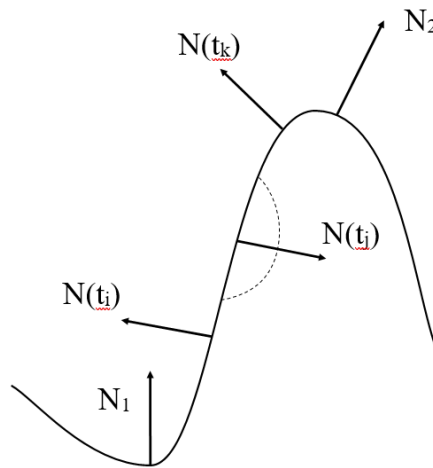
Рис. 11. Инвертирование нормали. Пунктиром — область, где нормаль инвертирована
