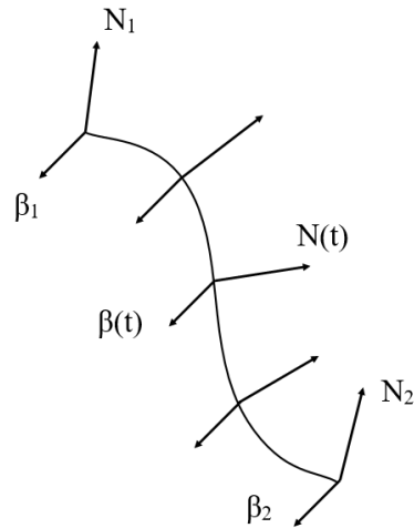
Рис. 12. Сравнение изменения интерполируемой нормали и бинормали на кривой
