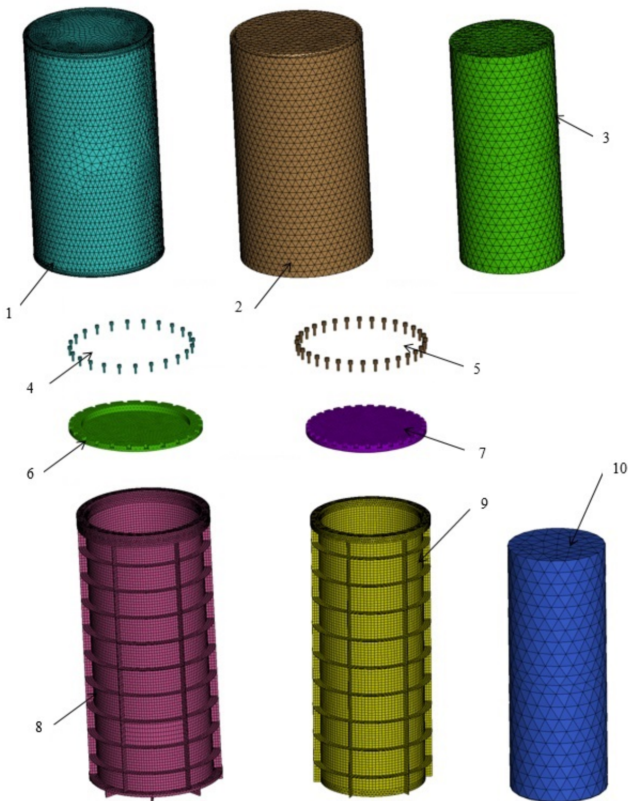
1 — наружная обечайка контейнера; 2 — перлитобетон контейнера; 3 — внутренняя обечайка контейнера; 4 — болты крепления наружной крышки; 5 — болты крепления внутренней крышки; 6 — крышка наружная; 7 — крышка внутренняя; 8 — емкость наружная; 9 — емкость внутренняя; 10 — корзины
