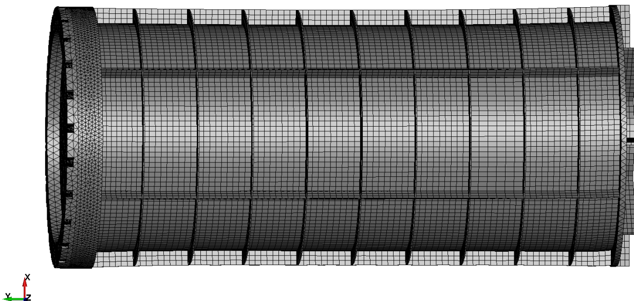
Рис. 7. Схема деформирования корпуса наружной емкости после падения на образующую
