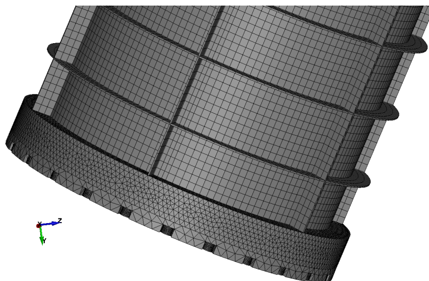
Рис. 4. Схема деформирования пенала ТУК-27/1 после падения на кромку крышки
