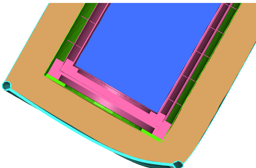
Рис. 3. Схема деформирования ТУК-27/1 после падения на кромку крышки
