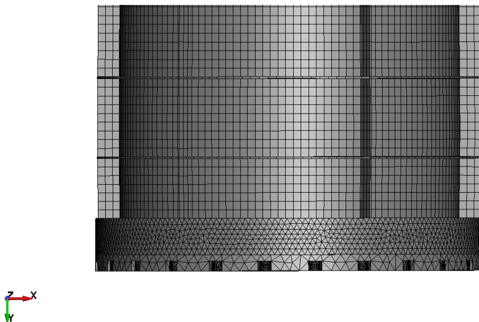
Рис. 5. Схема деформирования пенала ТУК-27/1 после падения на крышку
