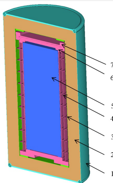
1 — наружная обечайка контейнера; 2 — перлитобетон контейнера; 3 — внутренняя обечайка контейнера; 4 — пенал; 5 — содержимое пенала; 6 — крышка пенала внутренняя; 7 — крышка пенала наружная
