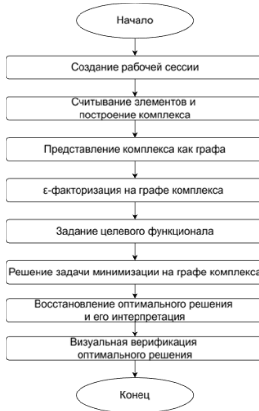
Рис. 2. Блок-схема программной платформы минимизации функционала на комплексах элементов
