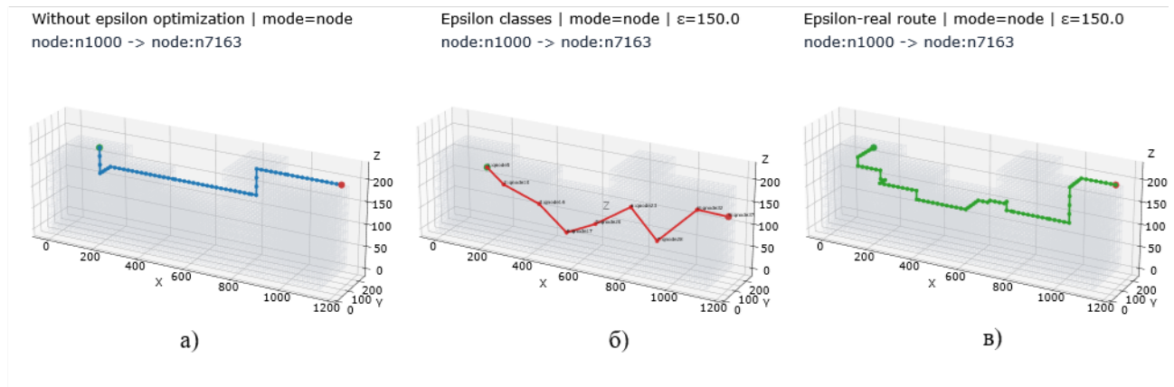
Рис. 3. Маршрут из узла n1 в узел n7163 : а) простой маршрут; б) факторизованный маршрут; в) лексикографический маршрут
