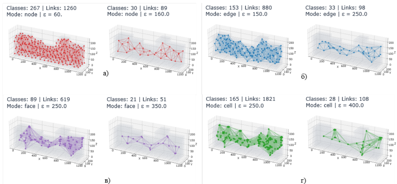
Рис. 1. Факторизация полиэдрального комплекса для элементов:
