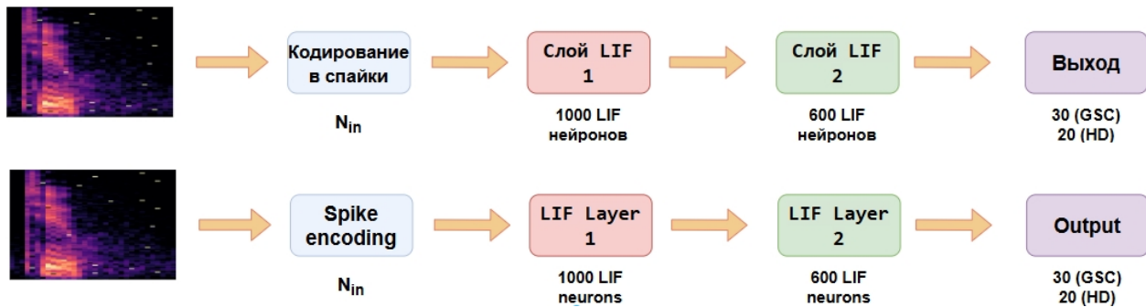
Рис. 3. Схема архитектуры MLP-LIF: спектрограмма, кодирование, два скрытых слоя LIF и выходной слой классификатора
